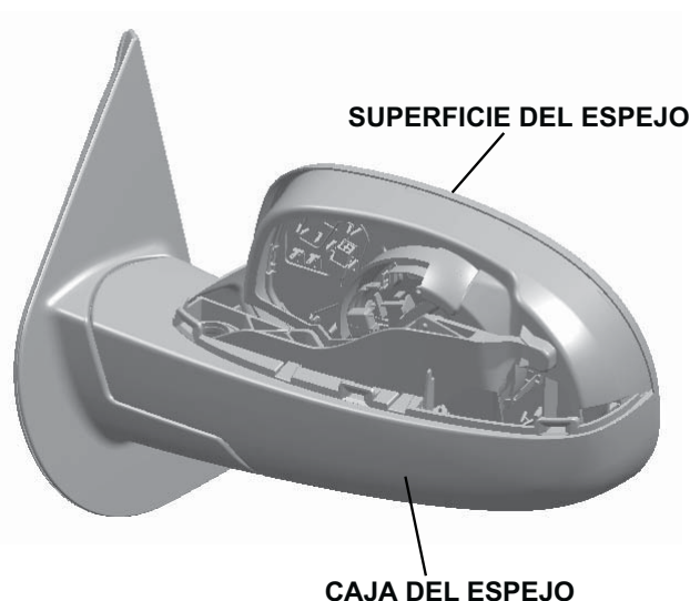
FIGURA 3A – Caja del espejo sin cubierta
